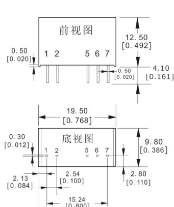
封装尺寸图
