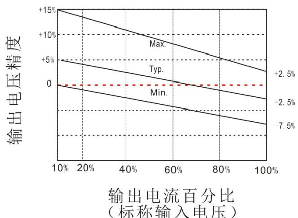
3. 3/5VDC输出 误差包络曲线图
